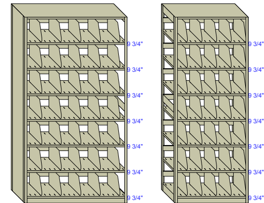
R4 42"W x 12"D H=76 1/4"
